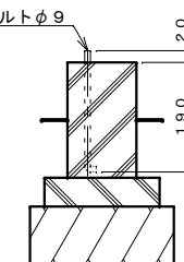
アンカーボルト埋設図 S=1:10
