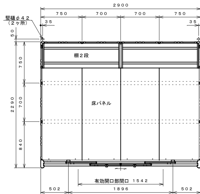
平面図 S=1:30
