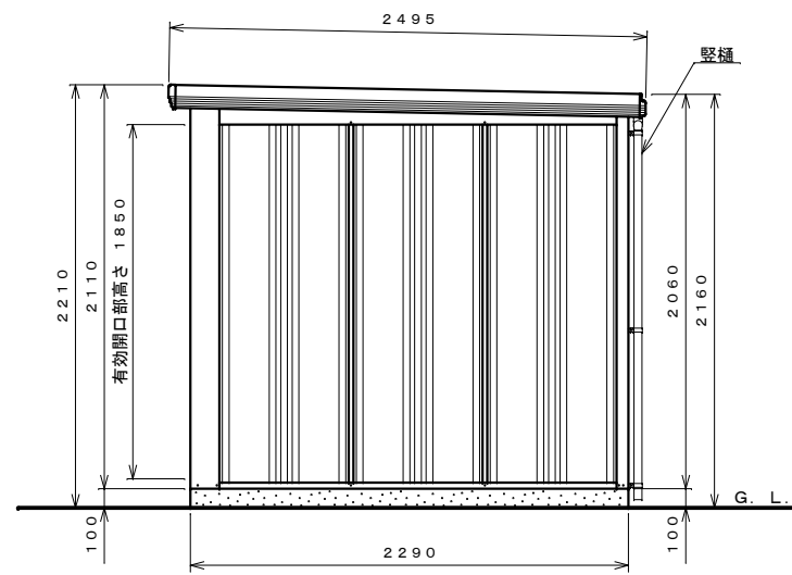
側面図 S=1:30
