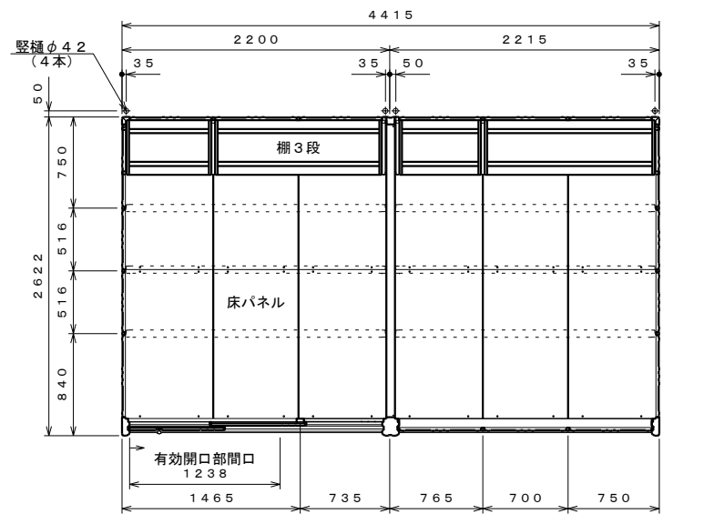
平面図 S=1:40
