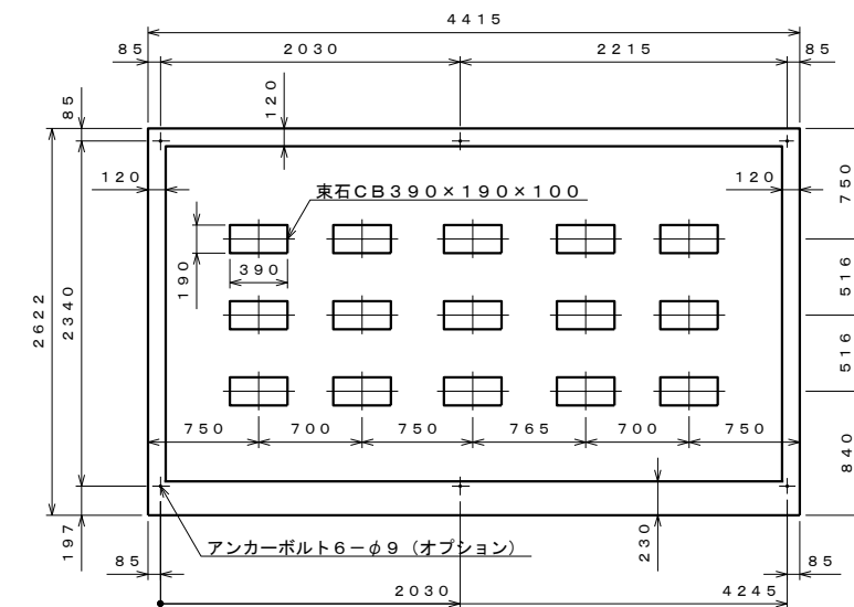
基礎伏せ図 S=1:40
