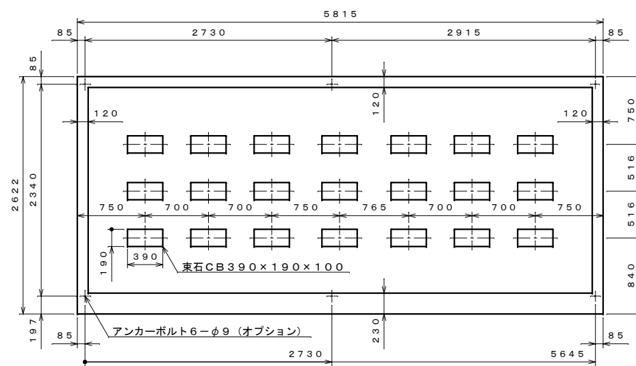
基礎伏せ図 S=1:40
