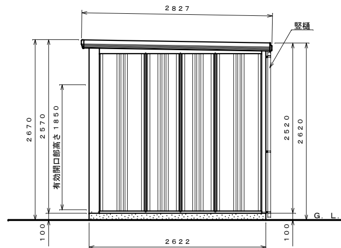
側面図 S=1:40
