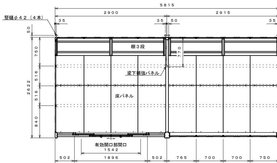
平面図 S=1:40
