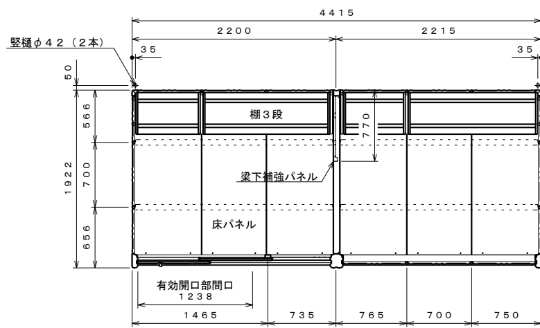
平面図 S=1:40
