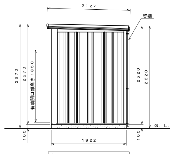
側面図 S=1:40
