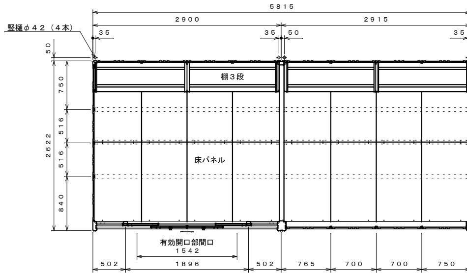
平面図 S=1:40
