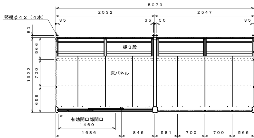
平面図 S=1:40
