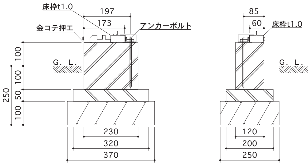
A-A断面図
