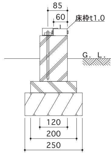
B-B断面図
