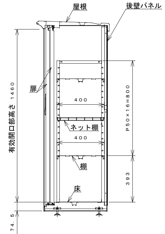
側面断面図
