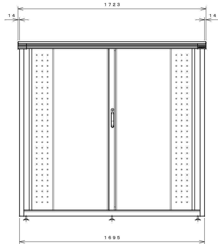
正面図
