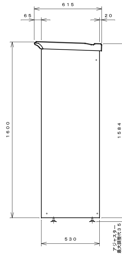
右側面図
