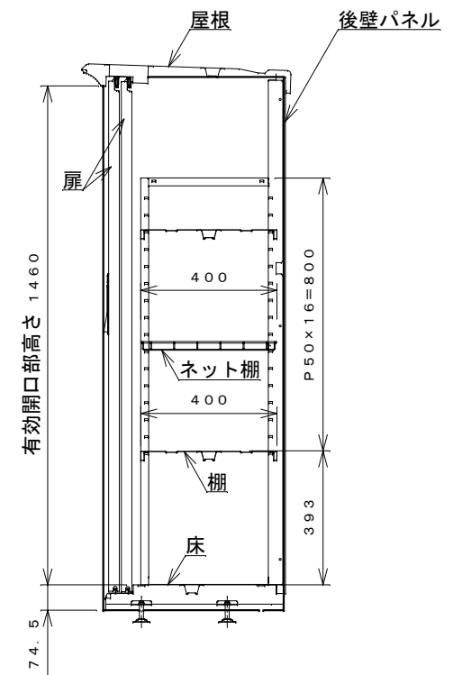
側面断面図
