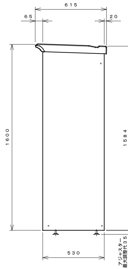
右側面図
