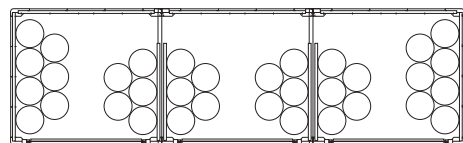
【50kg型容器参考収納例】
