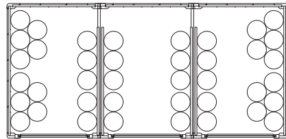
【50kg型容器参考収納例】
