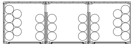
【50kg型容器参考収納例】
