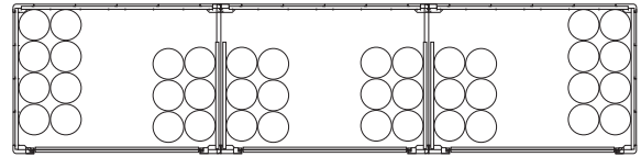
【50kg型容器参考収納例】
