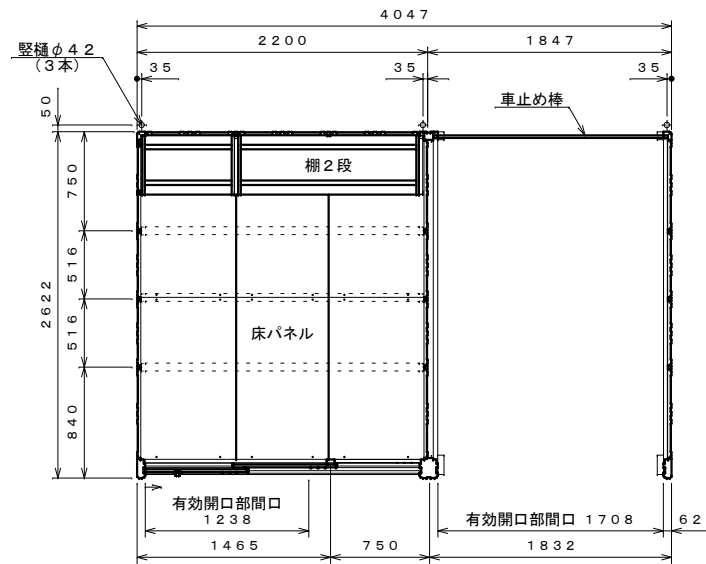
平面図 S=1:40
