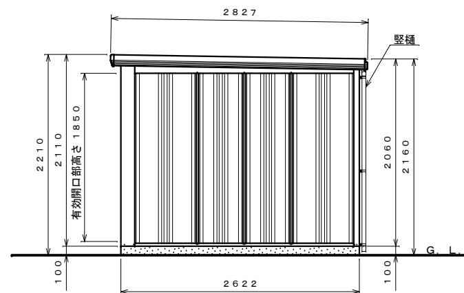
側面図 S=1:40
