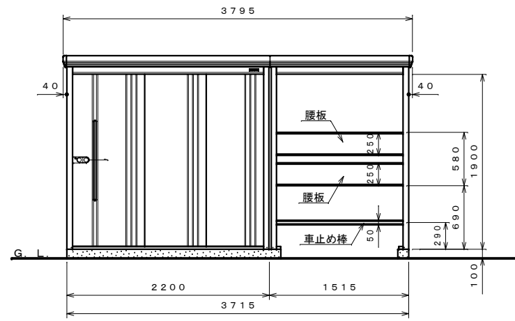
正面図 S=1:40
