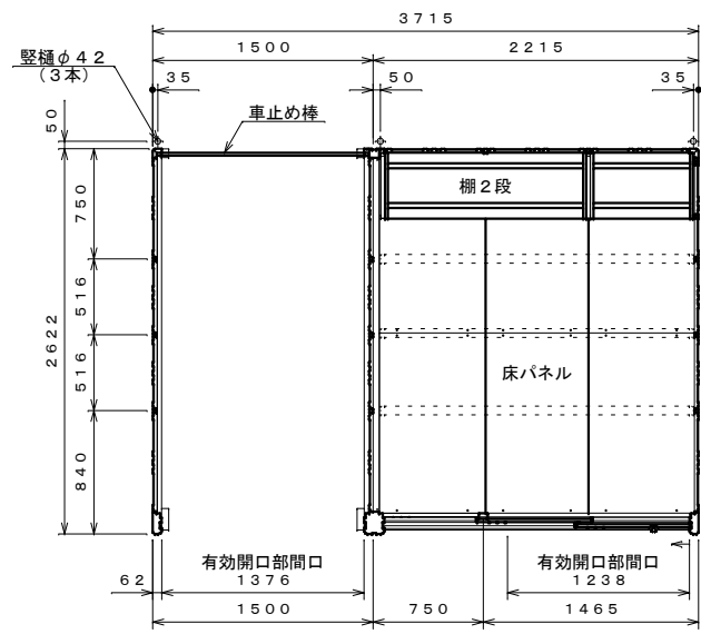
平面図 S=1:40
