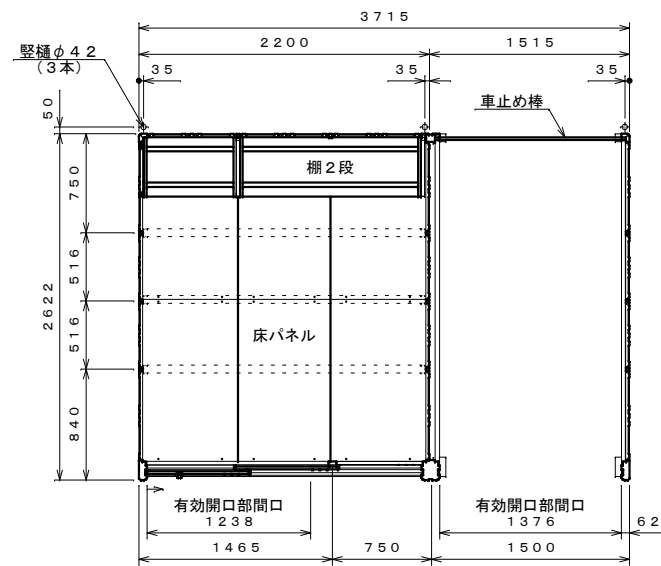
平面図 S=1:40
