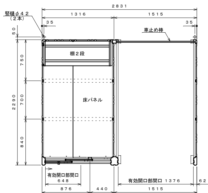
平面図 S=1:30
