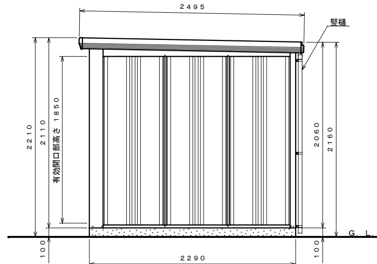
側面図 S=1:30
