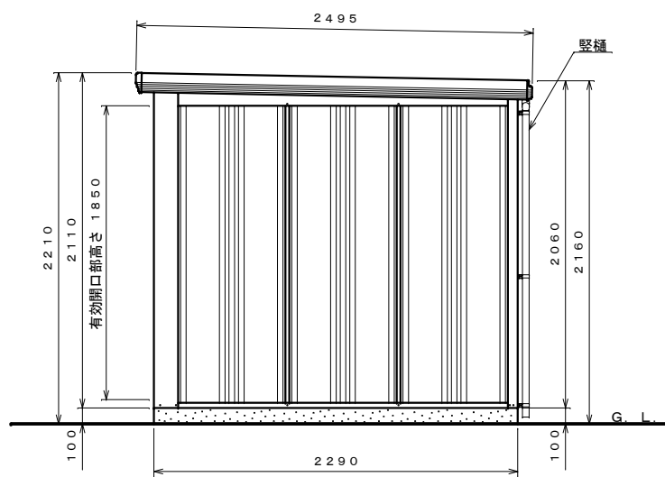
側面図 S=1:30
