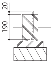
アンカー埋設図
