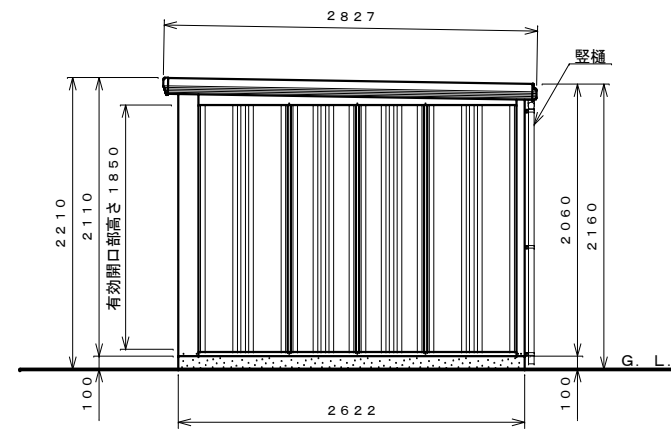
側面図 S=1:40
