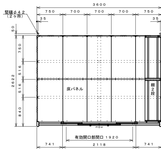
平面図 S=1:40
