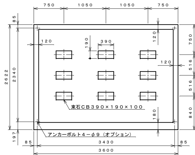
基礎伏せ図 S=1:40
