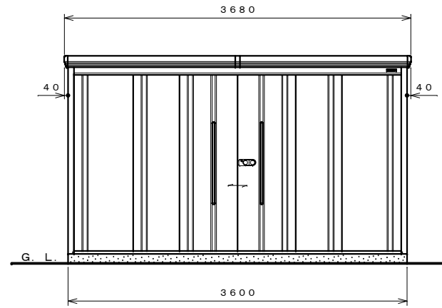
正面図 S=1:40
