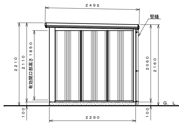
側面図 S=1:40
