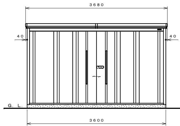
正面図 S=1:40
