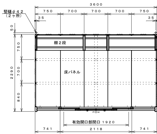
平面図 S=1:40
