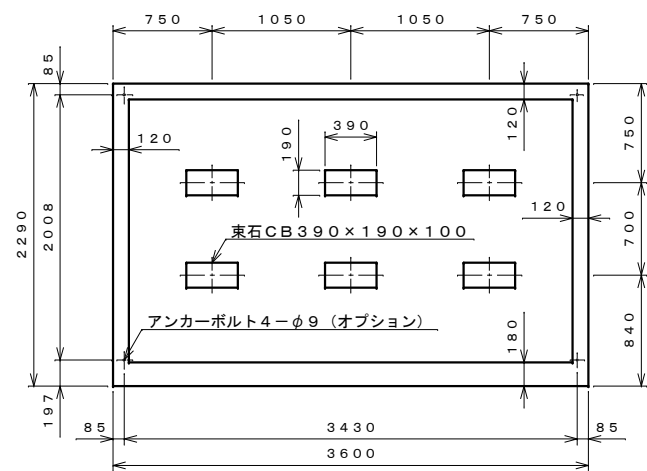
基礎伏せ図 S=1:40
