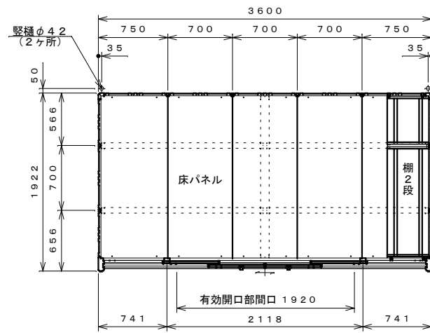
平面図 S=1:40
