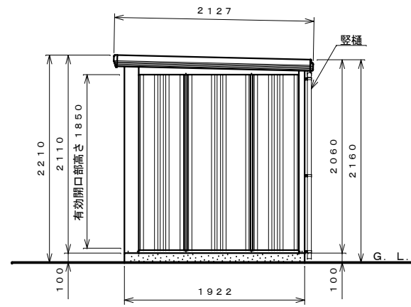
側面図 S=1:40
