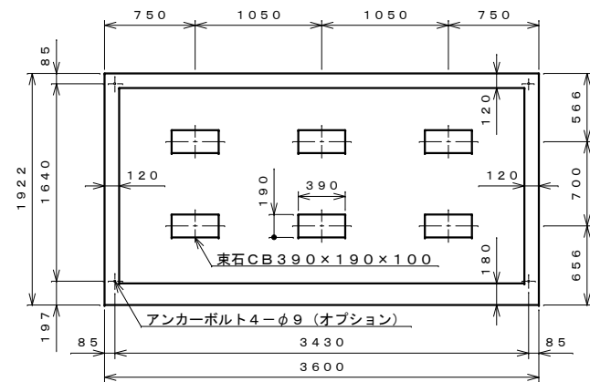
基礎伏せ図 S=1:40
