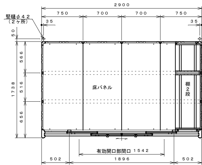
平面図 S=1:30
