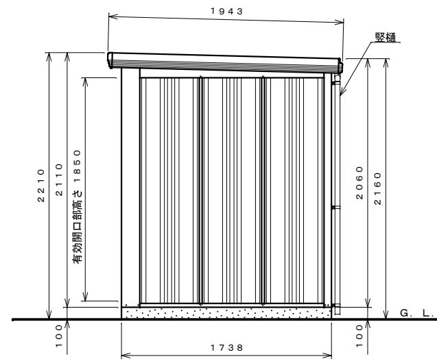
側面図 S=1:30
