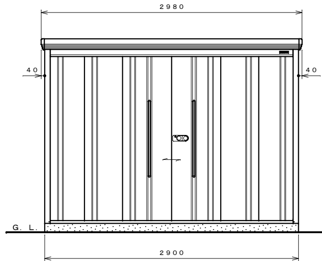
正面図 S=1:30
