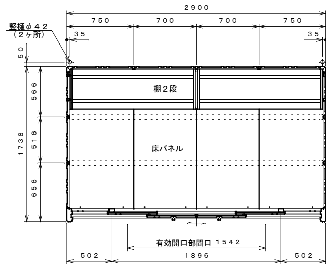
平面図 S=1:30
