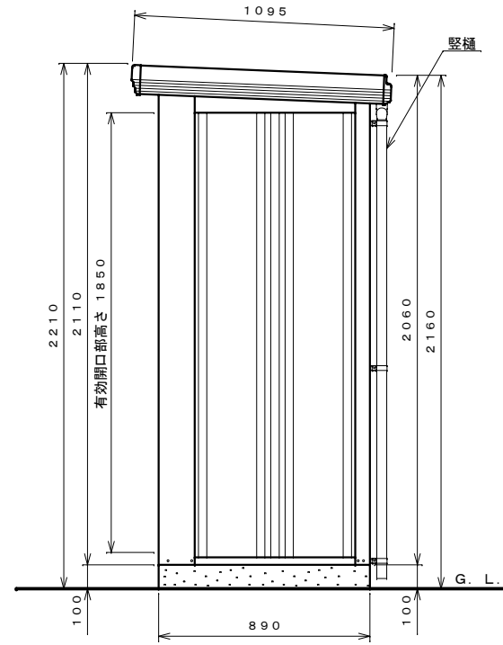
側面図 S=1:20
