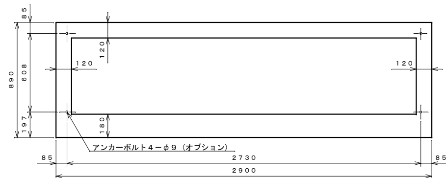
基礎伏せ図 S=1:20
