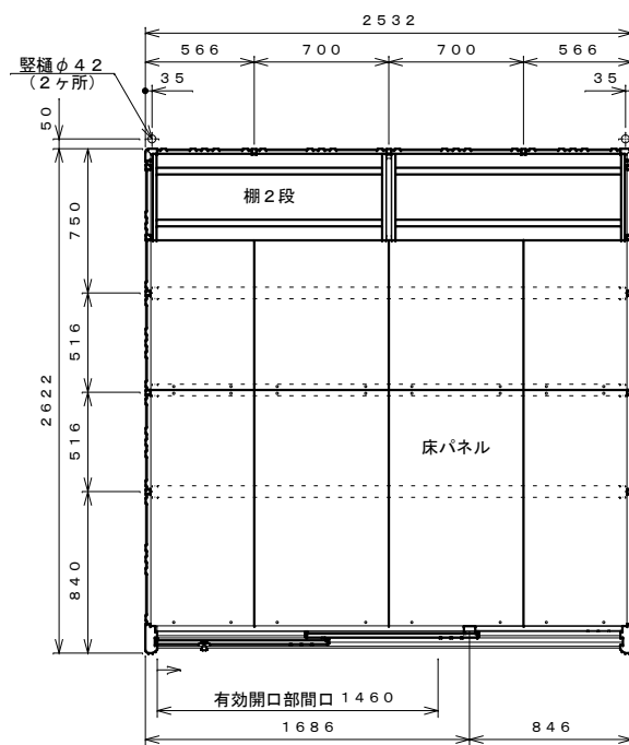
平面図 S=1:30
