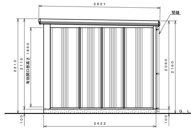
側面図 S=1:30
