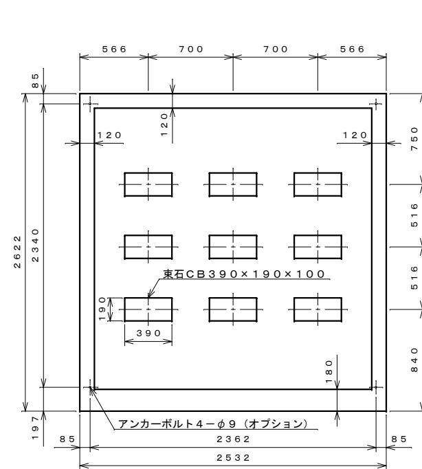
基礎伏せ図 S=1:30
