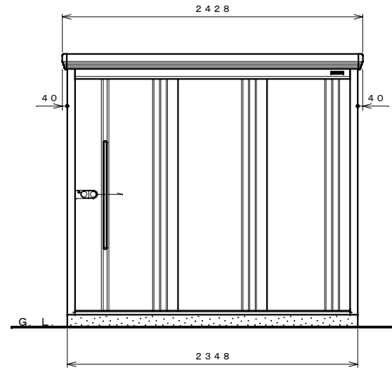
正面図 S=1:30
