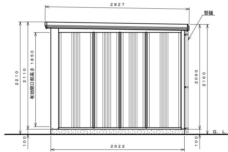
側面図 S=1:30
