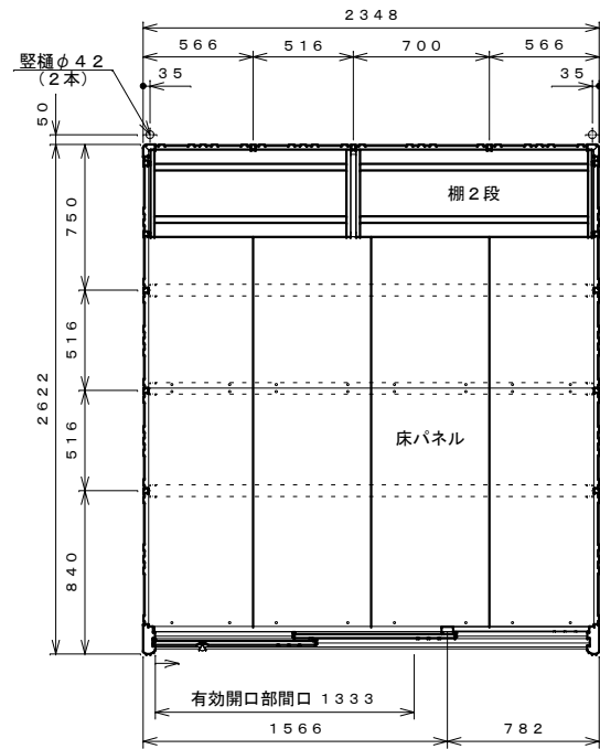
平面図 S=1:30
