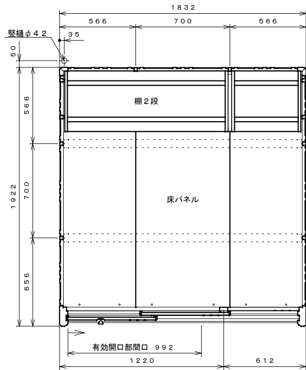
平面図 S=1:20
