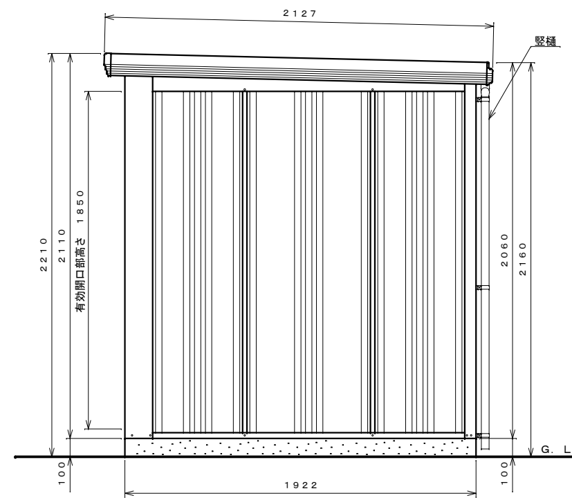
側面図 S=1:20
