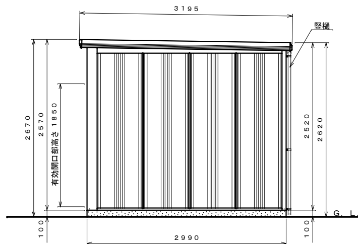
側面図 S=1:40
