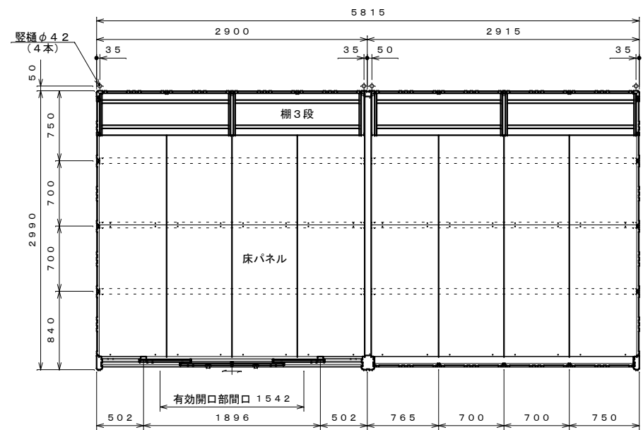
平面図 S=1:40
