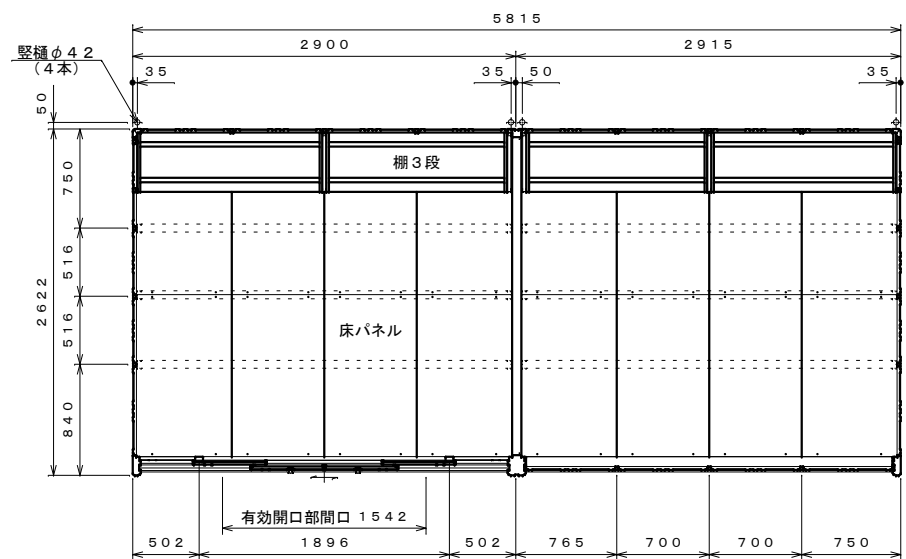
平面図 S=1:40
