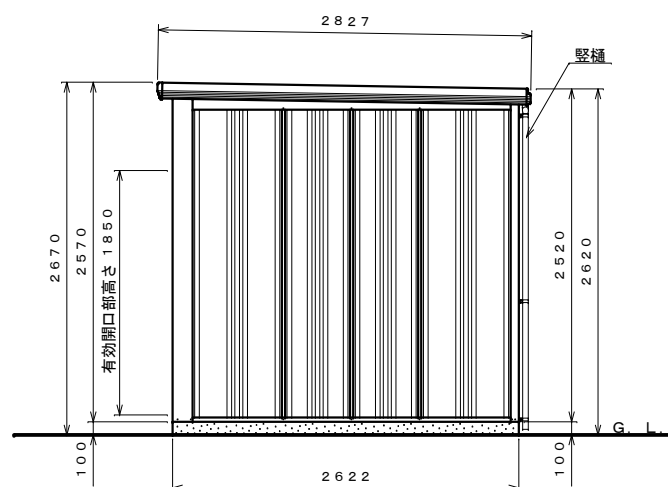
側面図 S=1:40
