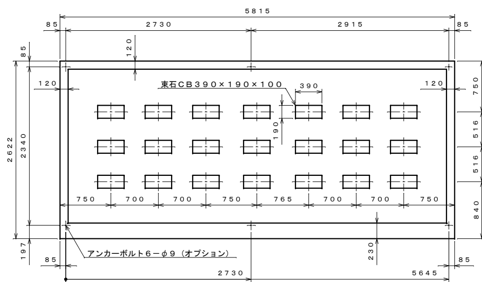
基礎伏せ図 S=1:40
