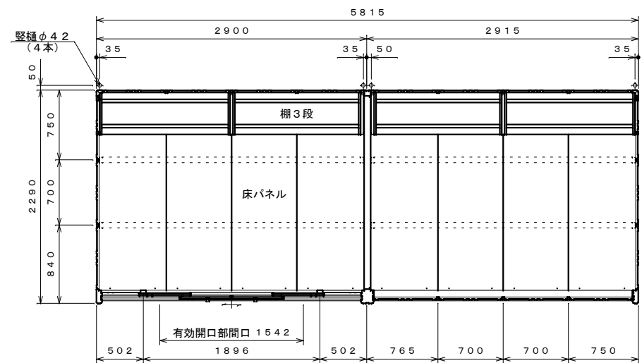
平面図 S=1:40
