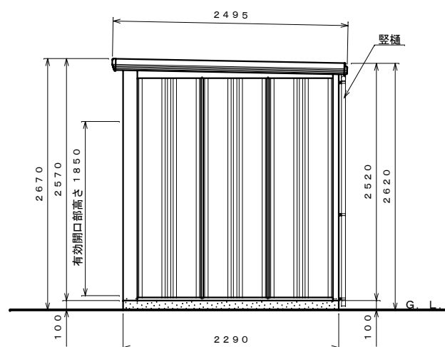
側面図 S=1:40
