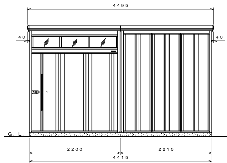
正面図 S=1:40
