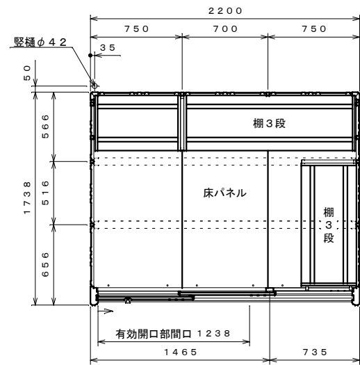
平面図 S=1:30
