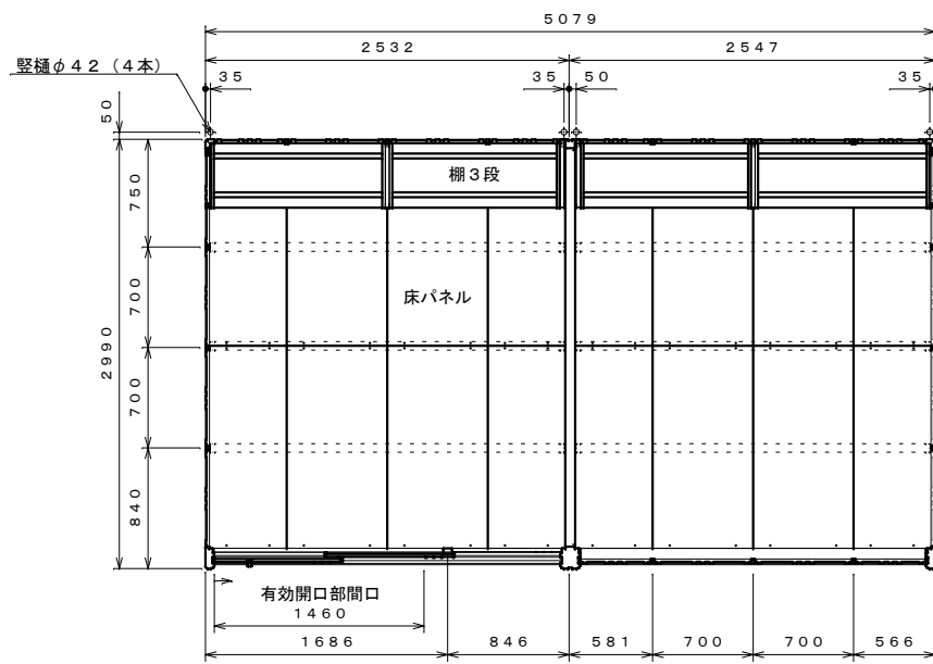
平面図 S=1:40
