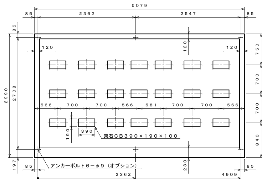
基礎伏せ図 S=1:40
