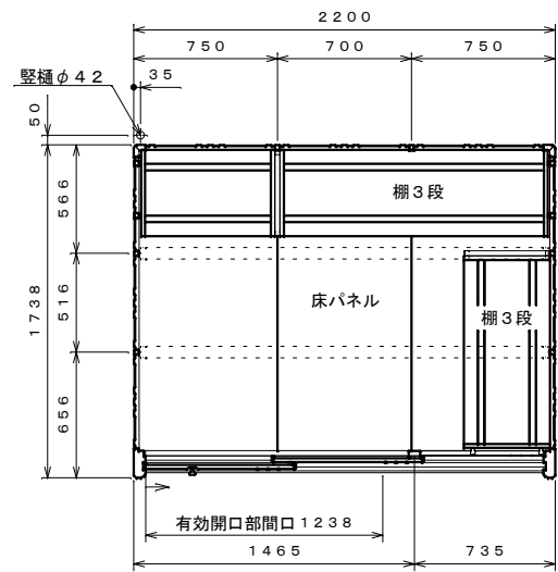
平面図 S=1:30
