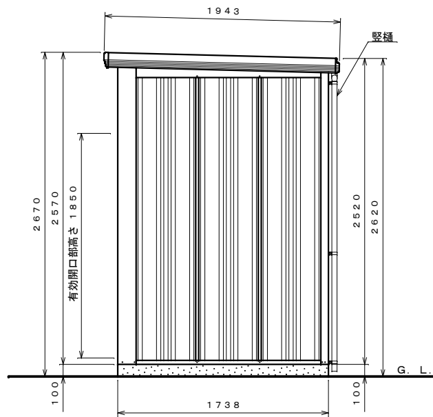
側面図 S=1:30
