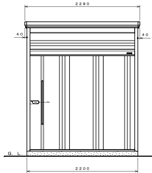
正面図 S=1:30
