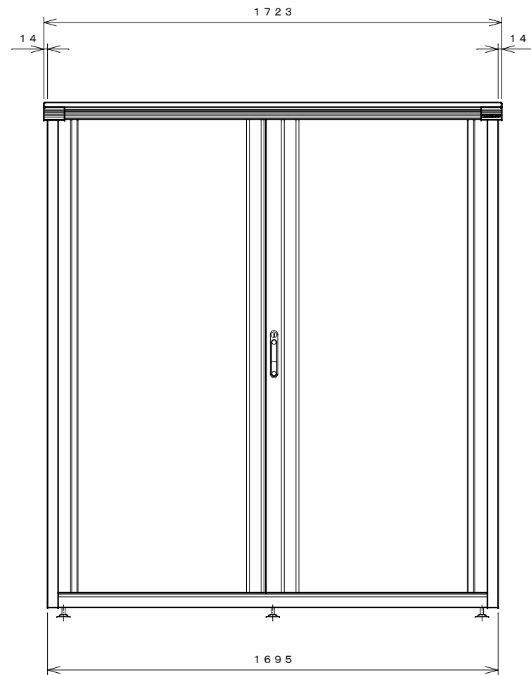
正面図
