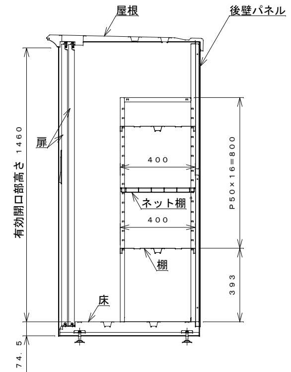
側面断面図
