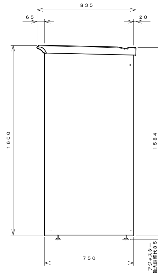
右側面図
