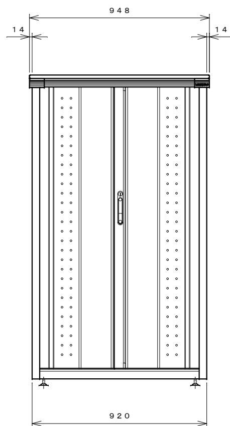
正面図
