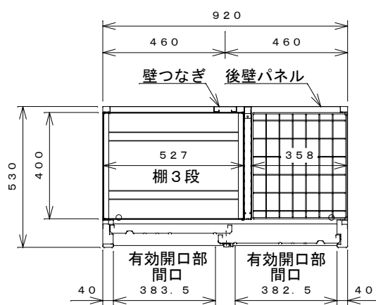
平面断面図
