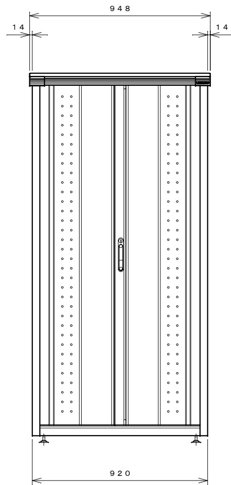
正面図
