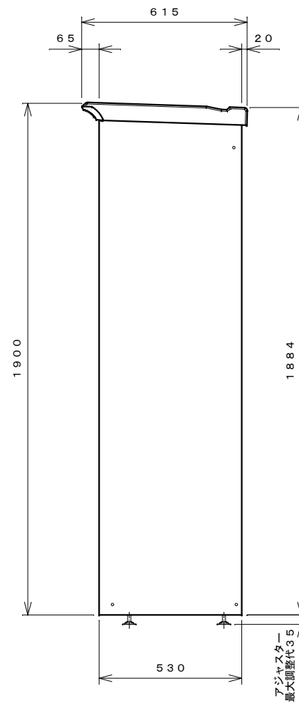
右側面図
