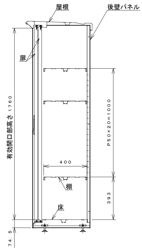
側面断面図
