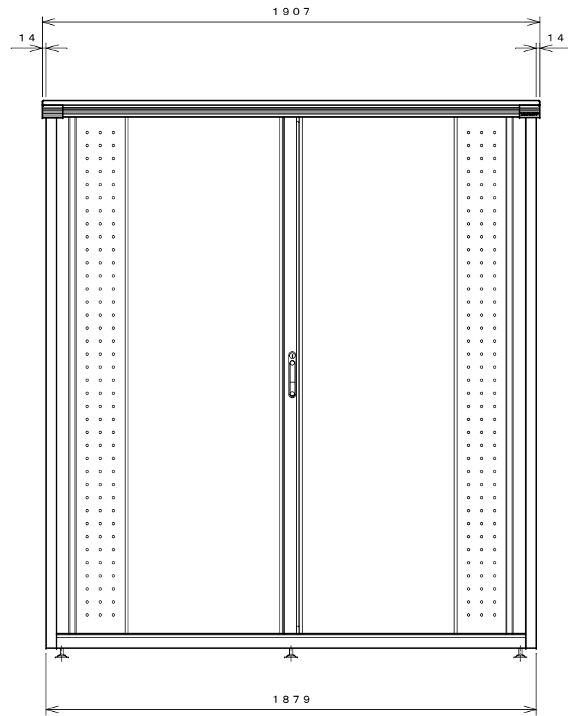
正面図
