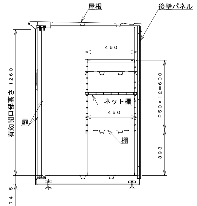
側面断面図
