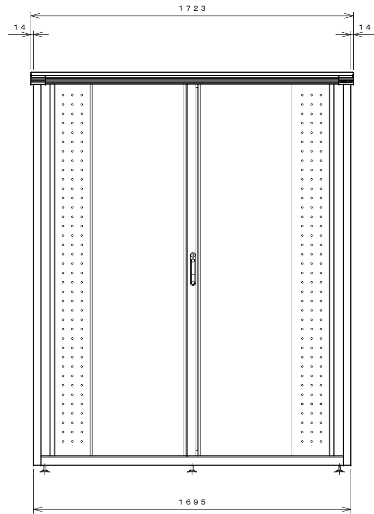
正面図
