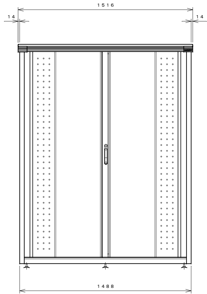
正面図
