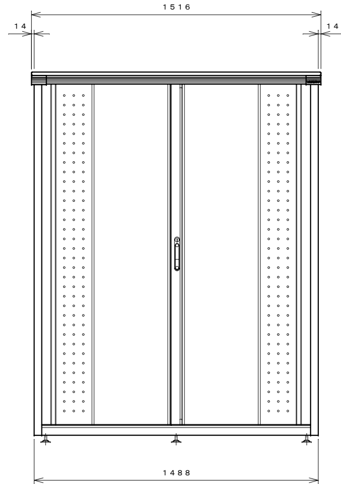
正面図
