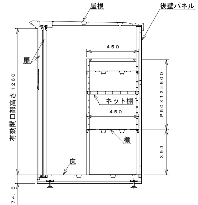
側面断面図
