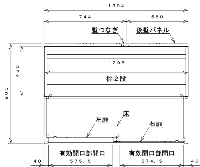
平面断面図
