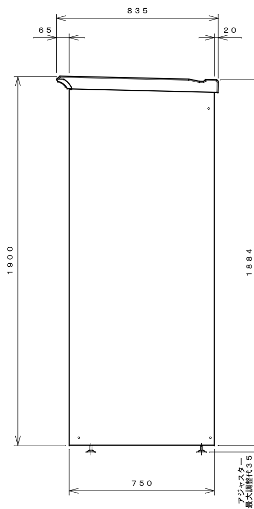
右側面図
