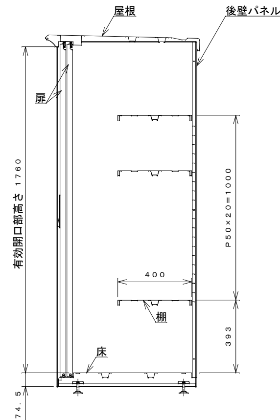
側面断面図
