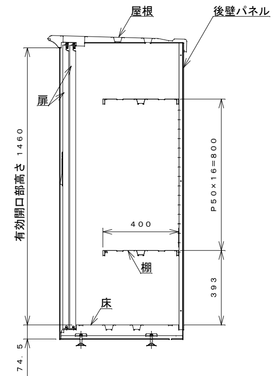
側面断面図
