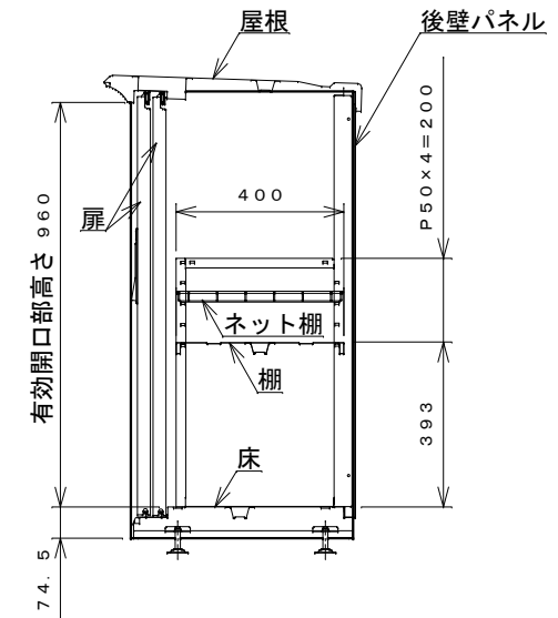
側面断面図
