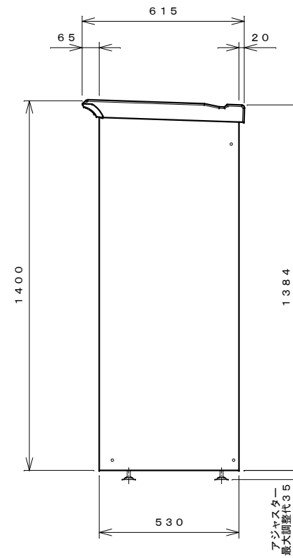
右側面図
