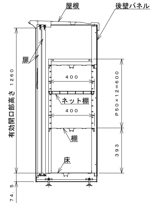
側面断面図
