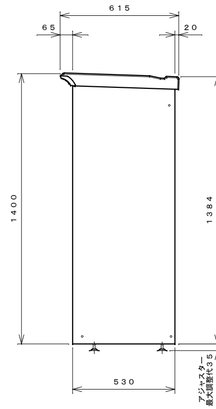
右側面図
