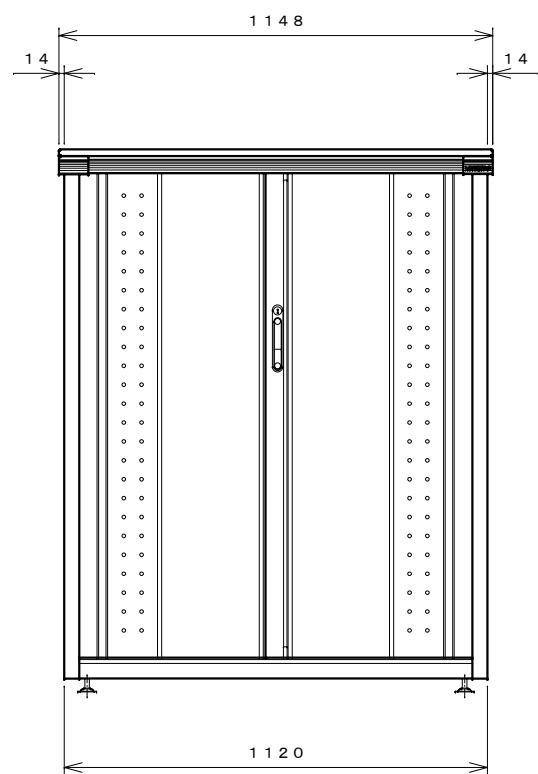
正面図
