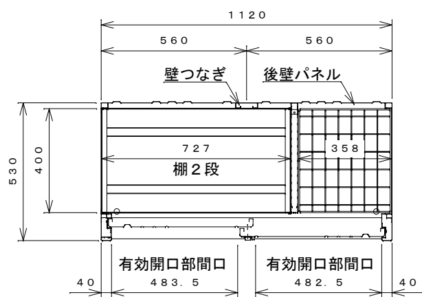
平面断面図
