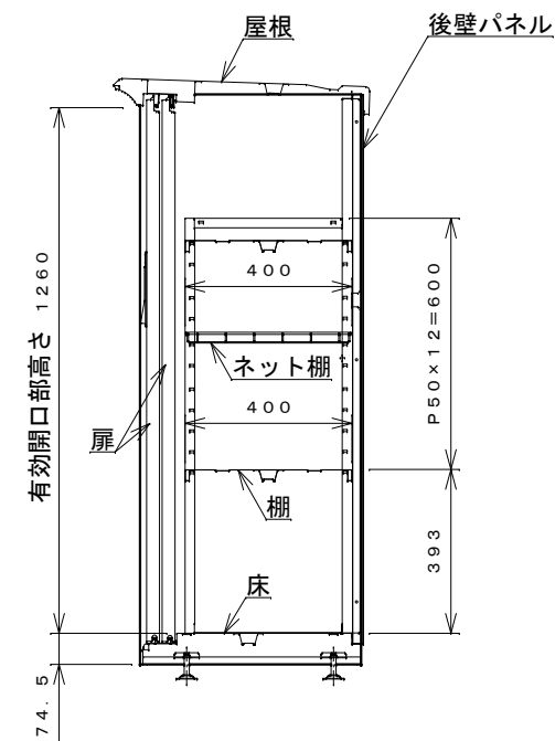
側面断面図
